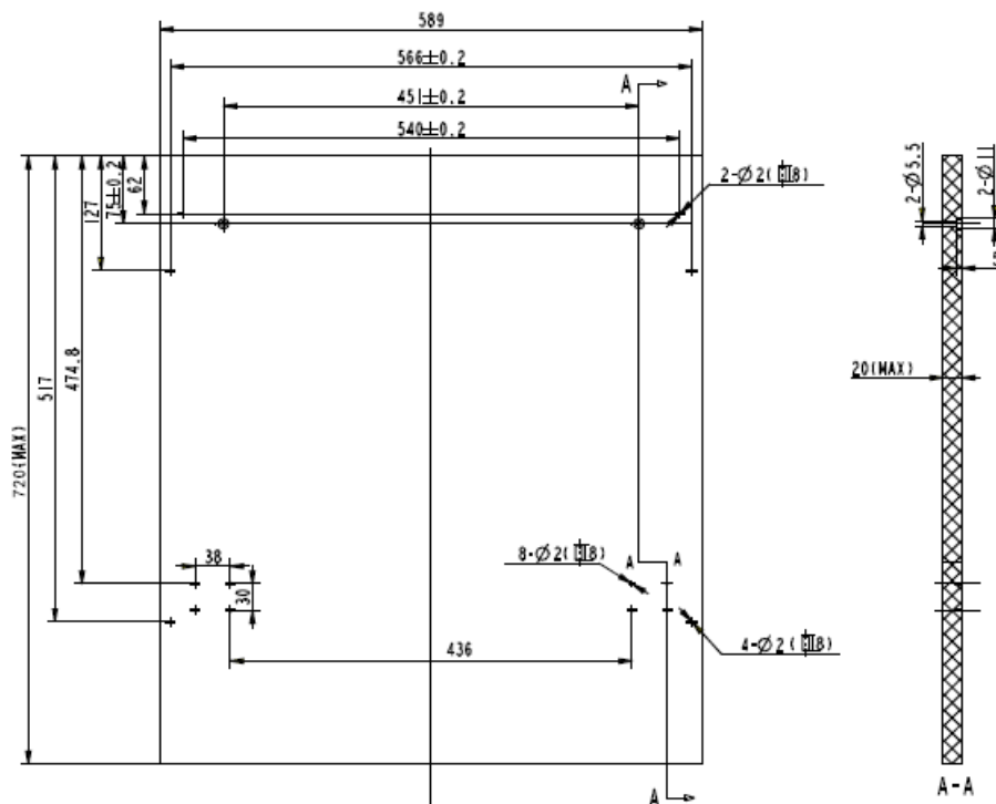
Декоративную панель следует устанавливать в соответствии с указанными на рисунке размерами.
