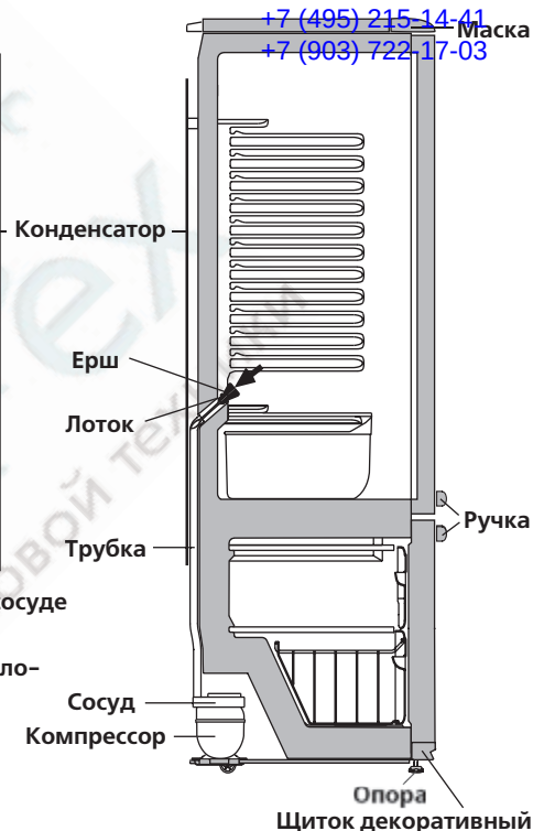
Рисунок 6 — Схема слива талой воды из холодильной камеры
