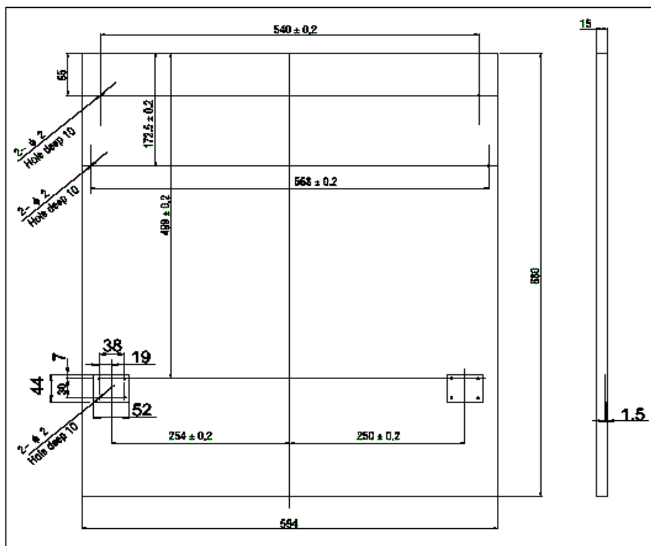
Рис. 3 Внешняя панель должна быть обработана согласно размеров на рисунке (размеры в мм).
