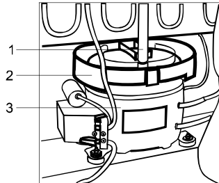
Рисунок Б.4 - Схема відведення талої води з холодильної камери Рисунок Б.4 - Схема отвода талой воды из холодильной камеры ნახაზი Б.4 - სამაცივრე კამერიდან გალღობილი წყლის გადმოსვლის სქემა Şəkil B. 4 - Soyuducu kameradan erimis suyun axma sxemi Б.4-сурет - Тоңазытқыш камерада еріген судың ағу сызбанұсқасы Figura B.4 – Schema scurgerii apei dezghețate din camera frigorifică B.4-rasm: Muz erishidan hosil bo'lgan suvni sovutish kamerasidan chiqarib tashlash chizmasi
