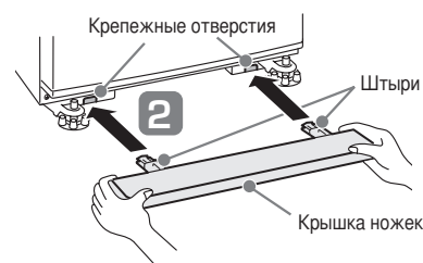
Крепежные отверстия
