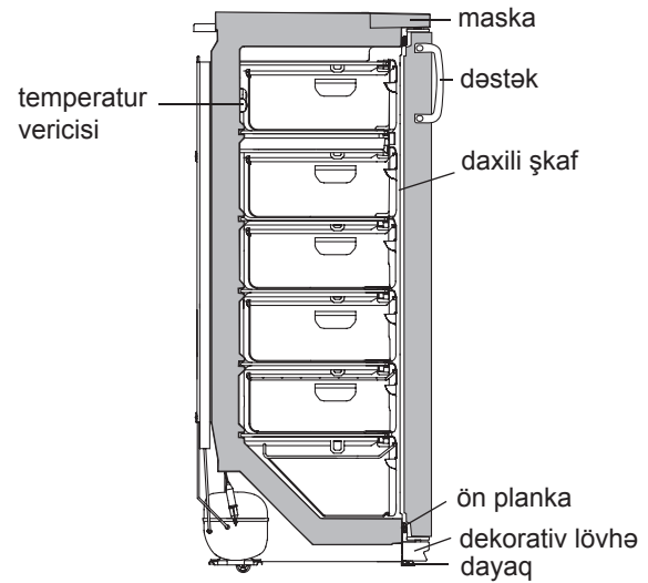
Şəkil 5 – Dondurucunun sxemi
