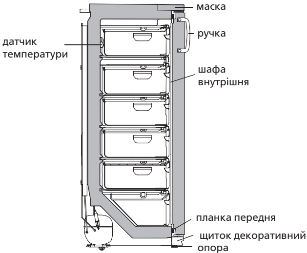
Рисунок 5 – Схема морозильника
