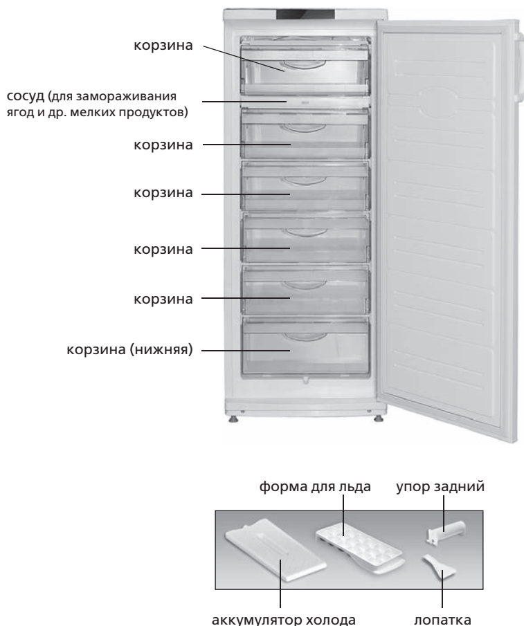
Рисунок 1 – Морозильник и комплектующие изделия
