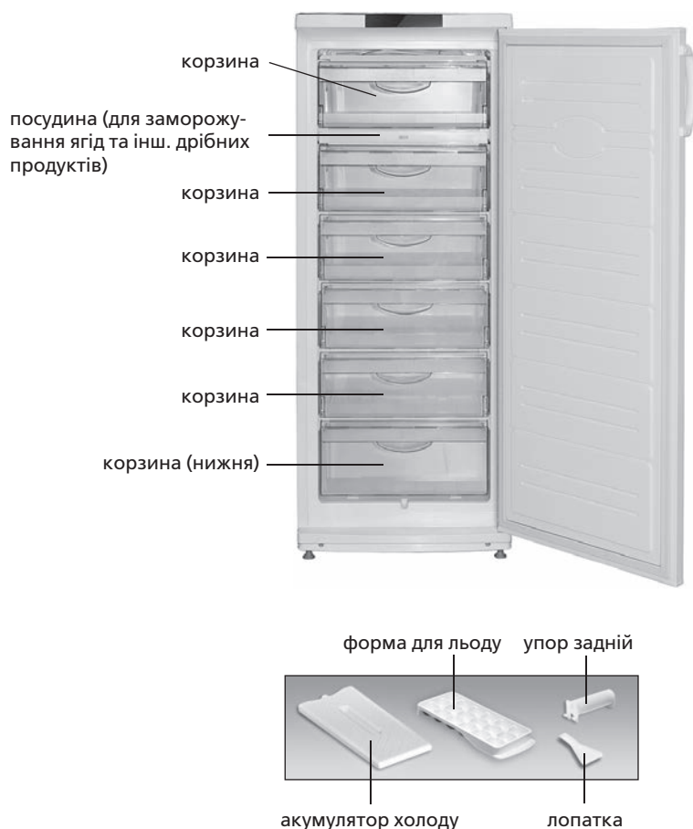
Рисунок 1 – Морозильник та комплектуючі вироби
