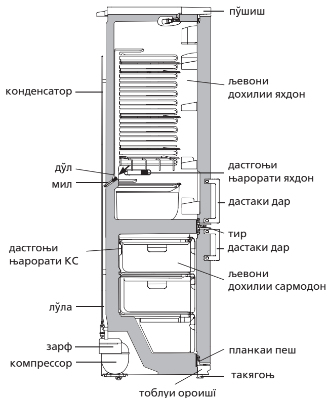
Расми 7 — Наќшаи партоби оби яхдон
