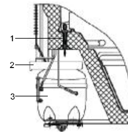
Рисунок Б.4 - Схема відведення талої води з холодильної камери/ Рисунок Б.4 - Схема отвода талой воды из холодильной камеры/ ნახაზი Б.4 - სამაცივრე კამერიდან გალღობილი წყლის გადმოღვრის სქემა/ Şekil B. 4 - Soğuducu kameradan erimiş suyun axma sxemi/ Б.4-сурет - Тоңазытқыш камерада еріген судың ағу сызбанұсқасы / Figura B.4 – Schema scurgerii apei dezghețate din camera frigorifică/ B.4-rasm: Muz erishidan hosil bo'lgan suvni sovutish kamerasidan chiqarib tashlash chizmasi.
