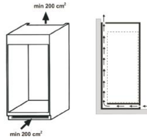
Рисунок Б.3 - Схема циркуляції повітря навколо холодильного приладу
