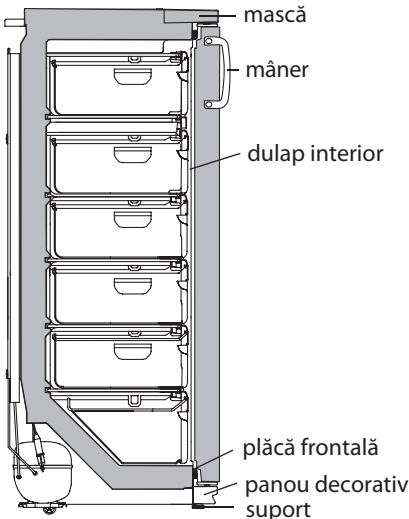
Figura 6 – Schema congelatorului
