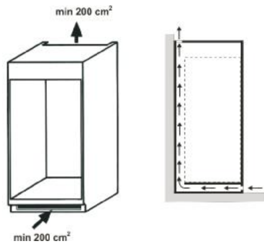
Рисунок Б.4 - Схема циркуляції повітря навколо холодильного приладу Рисунок Б.4 - Схема циркуляции воздуха вокруг холодильного прибора
