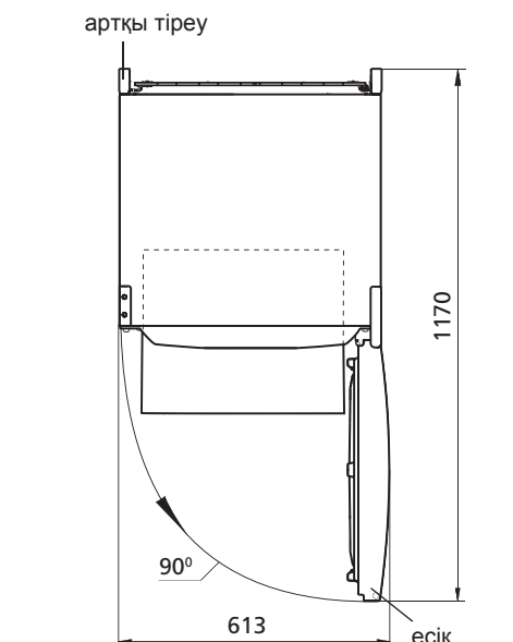
2 сурет — Тоңазытқыш (үстінен қарағанда)
