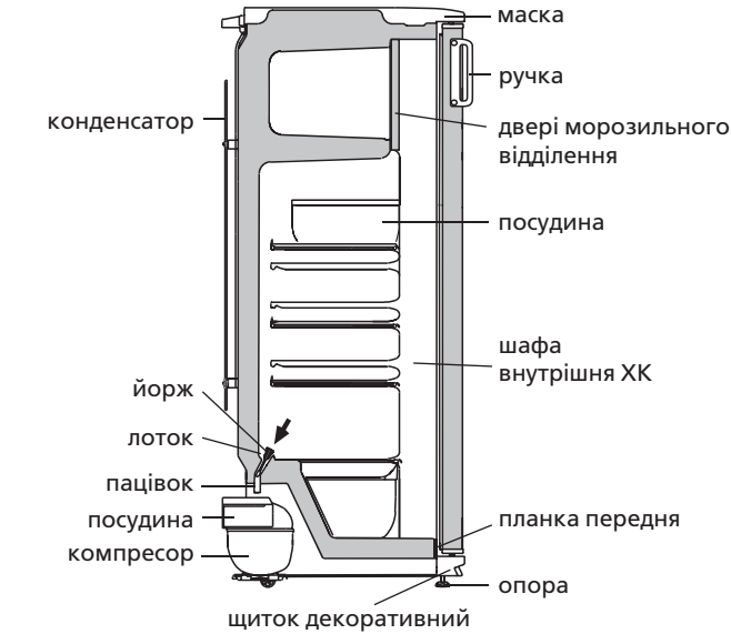
Рисунок 4 — Схема зливу талої води із ХК
