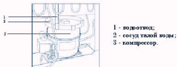
Рисунок Б.3 - Схема отвода талой воды из холодильной камеры
