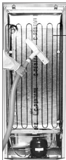
Конденсатор
