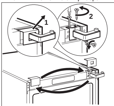
13. Установите верхнюю петлю на противоположной стороне прибора, а затем установите все крышки верхней петли.
