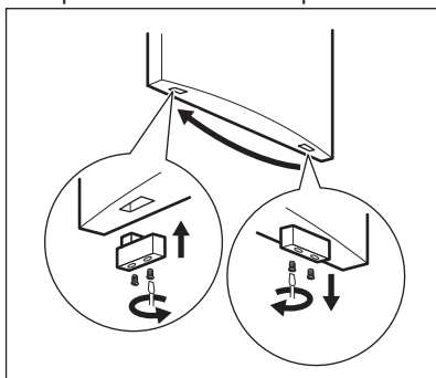
12. Снимите крышку верхней петли и отвинтите петлю от прибора.
