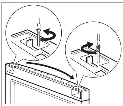
11. Снимите нижний ограничитель и установите его на противоположной стороне.
