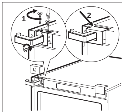
14. Осторожно установите верхнюю дверцу на среднюю петлю, затем продолжив установку дверцы с использованием верхней петли.
