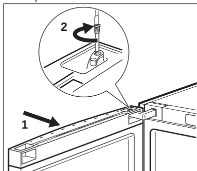
16. Установите на место крышку верхней дверцы.
