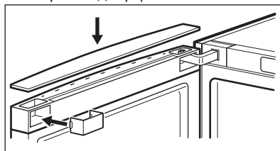
17. Привинтите ручки дверцы и заглушки на противоположной стороне.
