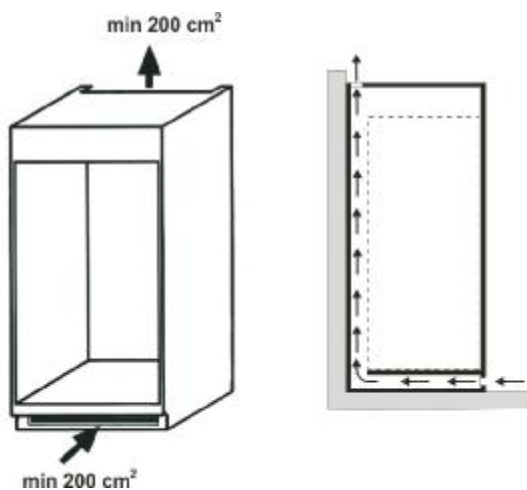
Рисунок Б.4 - Схема циркуляції повітря навколо холодильного приладу Рисунок Б.4 - Схема циркуляции воздуха вокруг холодильного прибора Şəkil B. 4. - Soyuducu cihazın ətrafında havanın dövriyyə sxemi ნახაზი Б.4 - სამაცივრე დანადგარის ირგვლივ ჰაერის ცირკულაციის სქემა Сурет Б.4- Тоңазытқыш прибор айналасындағы ауа айналысының схемасы
