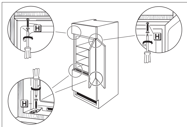
Соединить дверь прибора и дверь мебели
