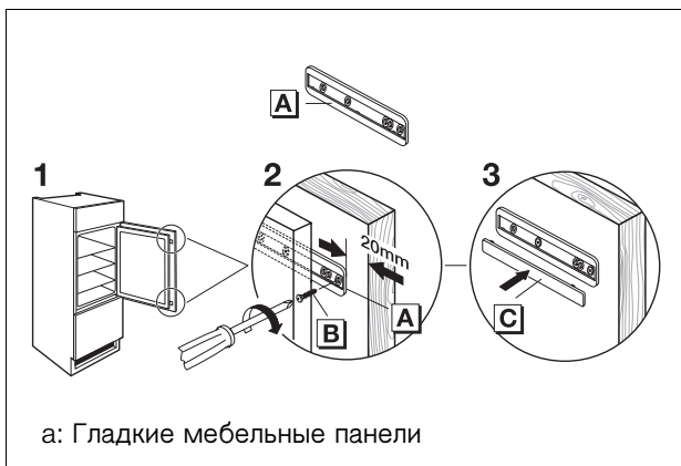
Соединить дверь прибора и дверь мебели
