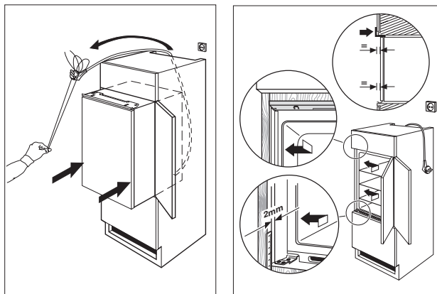
Привинтить прибор
