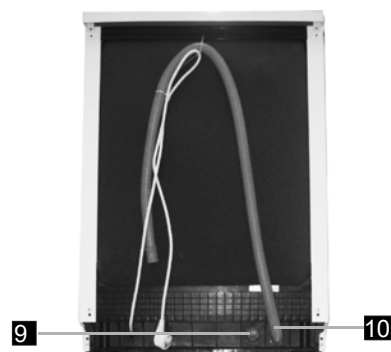
Вид сзади
