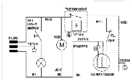
Схема электрическая принципиальная «BIRUSA V032»
