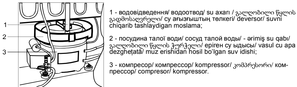
Рисунок Б.4 - Схема відведення талої води з холодильної камери
