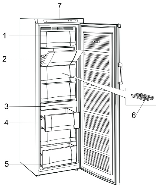
Рисунок Б.1 - Будова холодильника та розташування комплектуючих виробів Рисунок Б.1 - Устройство холодильника и расположение комплектующих изделий Şəkil B.1 - Soyuducu cihaz quruluşu və komplektə edici məmulatların (aksesuarların) yerləşməsi ნახაზი B.1 - მაგივარი და მავომპლექტებელი ნაწარმის განლაგება Б.1-сурет - Тоңазытқыштың құрылысы және кешендеуші бөлшектердің орналасуы Figura B.1 – Structura aparatului frigorific și amplasarea pieselor de completare B.1-rasm: Sovutgichning tuzilishi va butlovchi buyumlarning joylashishi.
