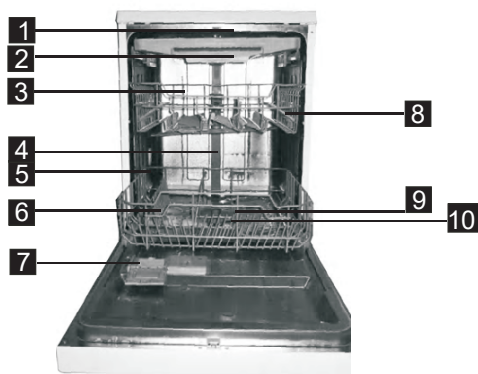
Вид спереди
