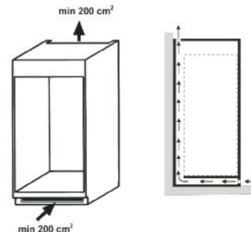
Рисунок Б.5 - Схема циркуляції повітря навколо холодильного приладу Рисунок Б.5 - Схема циркуляции воздуха вокруг холодильного прибора Şekil B. 5. - Soyuducu cihazın etrafında havanın dövrüyüş sxemi ნახაზი Б.5 - სამაცივრე დანადგარის ირგვლივ ჰაერის ცირკულაციის სქემა Сурет Б.5 - Тоңазытқыш прибор айналасындағы ауа айналысының схемасы Figura B.5 – Schema de circulație a aerului în jurul instalației frigorifice B.5-rasm: : Sovutish uskunasining atrofiga havo aylanish chizmasi
