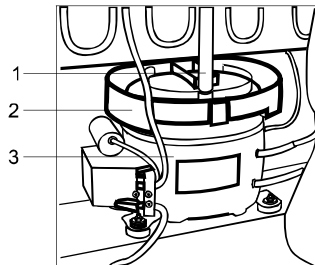
Рисунок Б.4 - Схема відведення талої води з холодної камери Рисунок Б.4 - Схема отвода талой воды из холодильной камеры ნახაზი Б.4 - სამაცივრე კამერიდან გაღლობილი წყლის გადმოსვლის სქემა Şəkil B. 4 - Soyuducu kameradan erimış suyun axma sxemi Б.4-сурет - Тоңазытқыш камерадаң еріген судың ағу сызбанұсқасы Figura B.4 – Schema scurgerii apei dezghețate din camera frigorifică B.4-rasm: Muz erishidan hosil bo'lgan suvni sovutish kamerasidan chiqarib tashlash chizmasi
