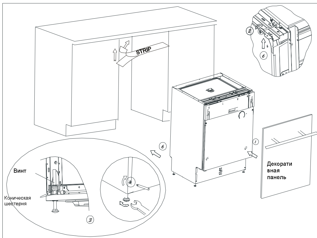
[Рис. 7] Порядок установки
