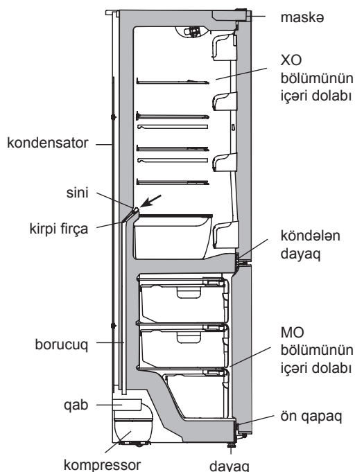
Rəsim 5 — XO bölümünün ərimiş axıntı sularının tökülməsi sxemi
