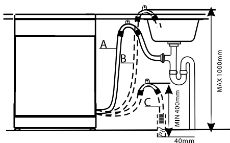
Рис. 6. Подсоединение сливного шланга
