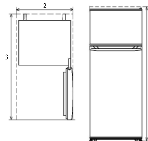
Рисунок Б.5 - Габаритный простір Рисунок Б.5 - Габаритное пространство Şəkil B. 5. - Qabarit space ნახაზი Б.5 - განზომილებიანი სივრცე Сурет Б.5 - Пішіндік кеңістік Figura B.5 – Dimensiuni de spațiu B.5-rasm: Габарит бұшлик
