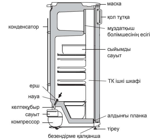
4 сурет — Еріген суды ТК-нан ағызу схемасы
