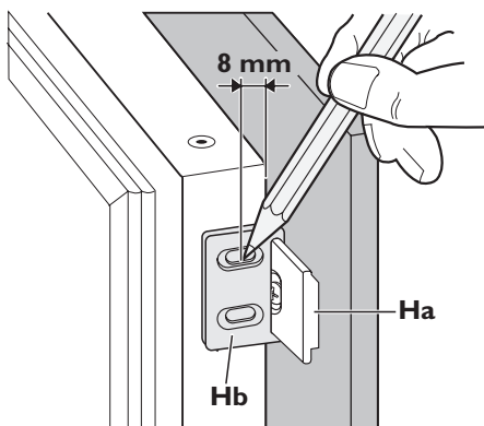
12. Снимите скобы и отметьте расстояние 8 мм от внешнего края дверцы для гвоздя (К).
