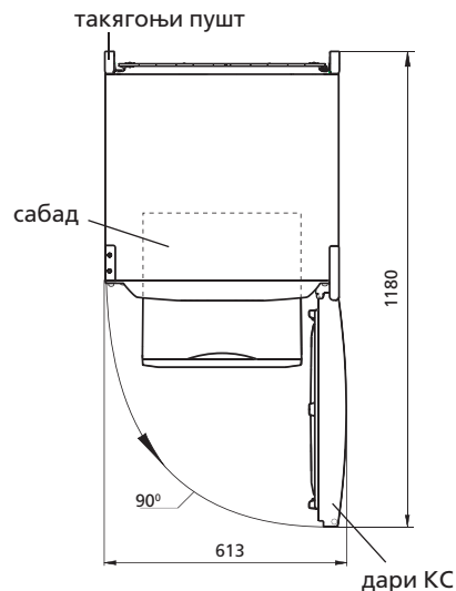
Расми 2 — Яхдон (намуди болої)
