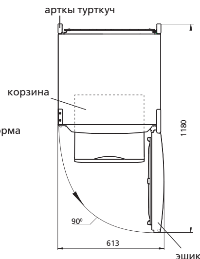
Сурот 2 — Муздаткыч (устунон корунушу)
