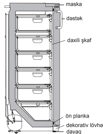
Şəkil 6 – Dondurucunun sxemi
