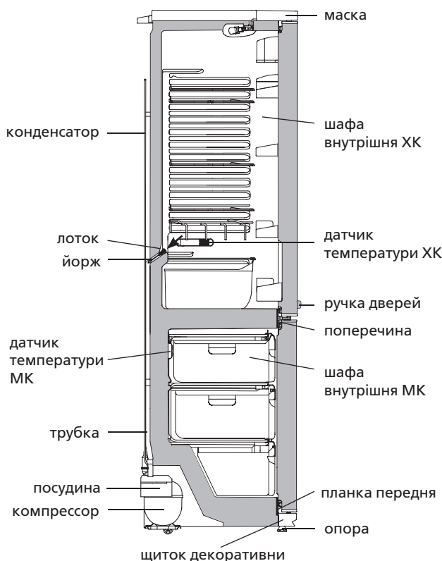
Рисунок 7 — Схема зливу талої води із ХК
