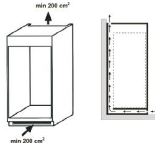
Рисунок Б.3 - Схема циркуляції повітря навколо холодильного приладу
