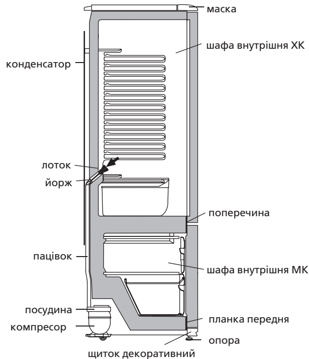
Рисунок 4 – Схема зливу талої води із ХК
