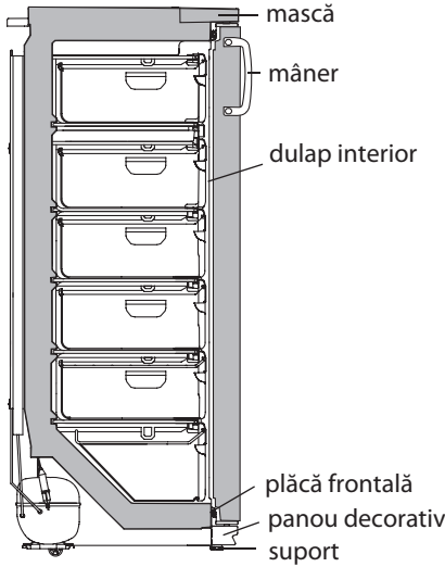
Figura 6 – Schema congelatorului
