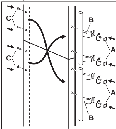
21. Привинтите ручки дверцы и заглушки на противоположной стороне.
