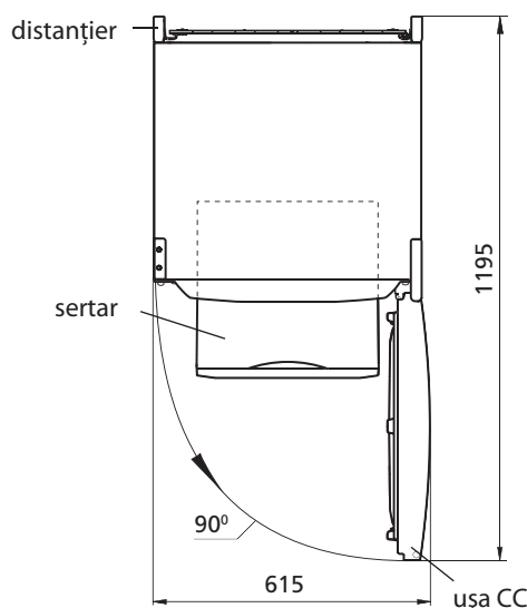
Figura 2 — Frigider (vederea de sus)
