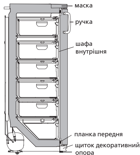
Рисунок 6 – Схема морозильника
