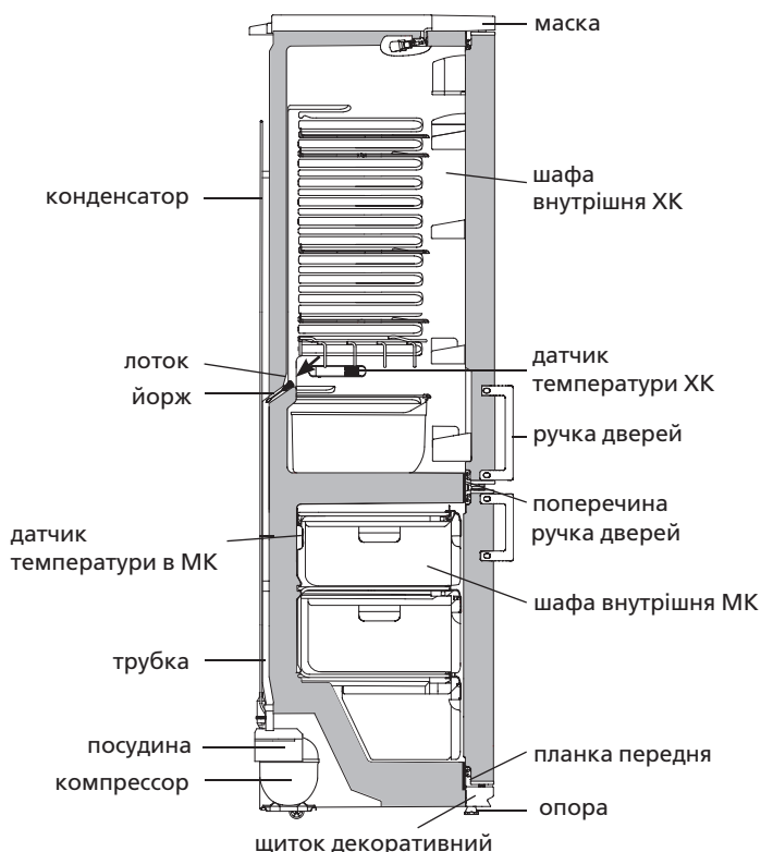
Рисунок 7 — Схема сливу талої води із ХК
