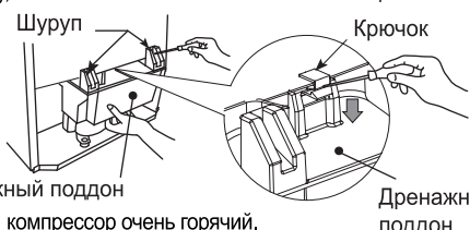
Дренажный поддон
