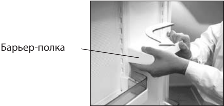
Рисунок 6 — Схема перенавески барьера-полки
