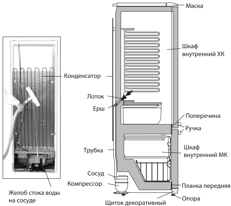
Рисунок 7 — Уборка холодильника (вид сзади)
