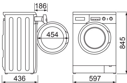
Размеры в миллиметрах
