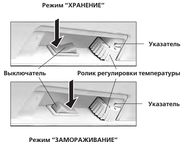
Рисунок 4 — Схема переключения режимов
