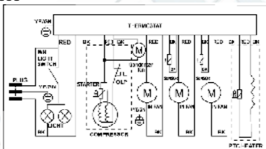
Схема электрическая принципиальная «BIRUSA VD45S»
