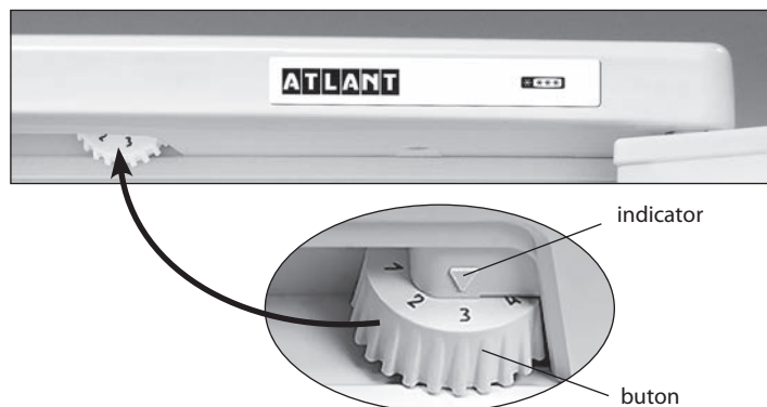
Figura 3 — Reglarea temperaturii
