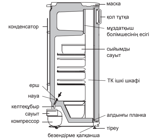
4 сурет — Еріген суды ТК-нан ағызу схемасы
