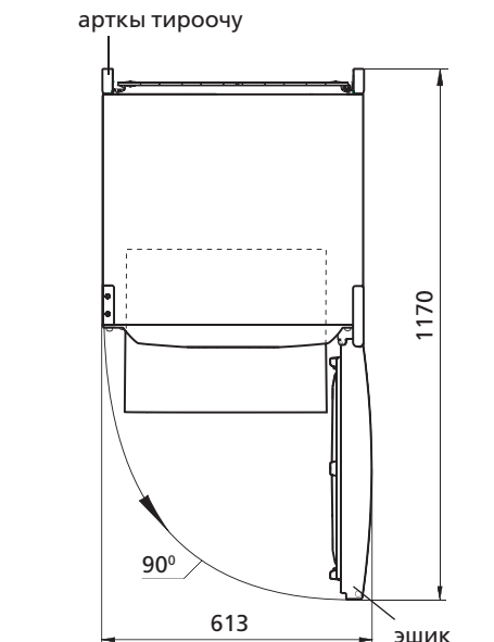
Сурот 2 — Муздаткыч (устунон корунушу)
