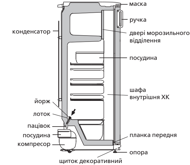
Рисунок 4 — Схема сливу талої води із ХК
