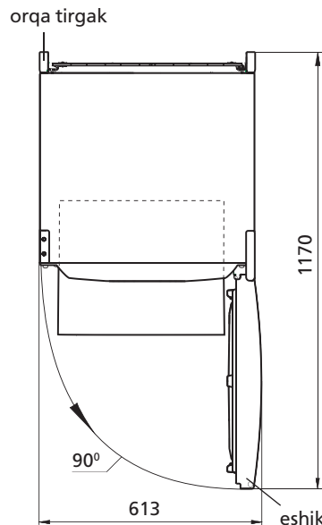
2 rasm — Sovutgich (tepadan ko'rinish)
