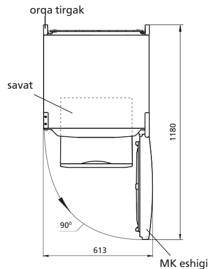
2 rasm - Sovutgich (tepadan ko'rinish)
